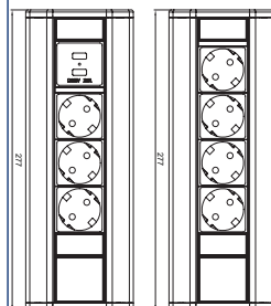
Rys.2 Wymiary techniczne
