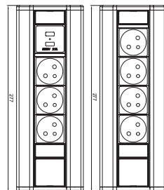
Rys.1 Wymiary techniczne
